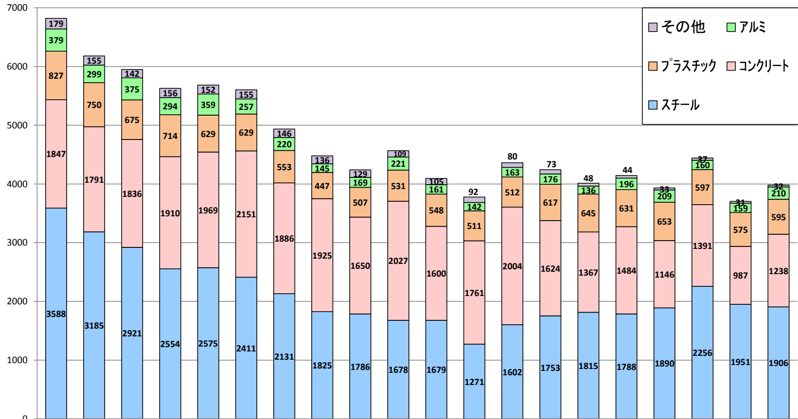
フリーアクセスフロアの材質別実績
