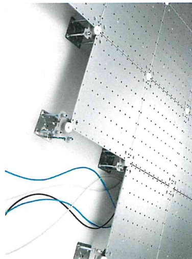
フリーアクセスフロアLAF-T500
